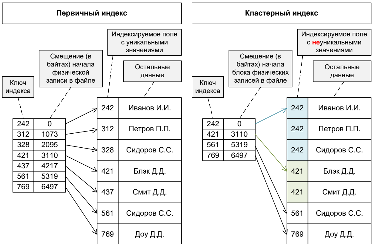
Рисунок 2.4.с — Схематичное представление первичного и кластерного индекса
