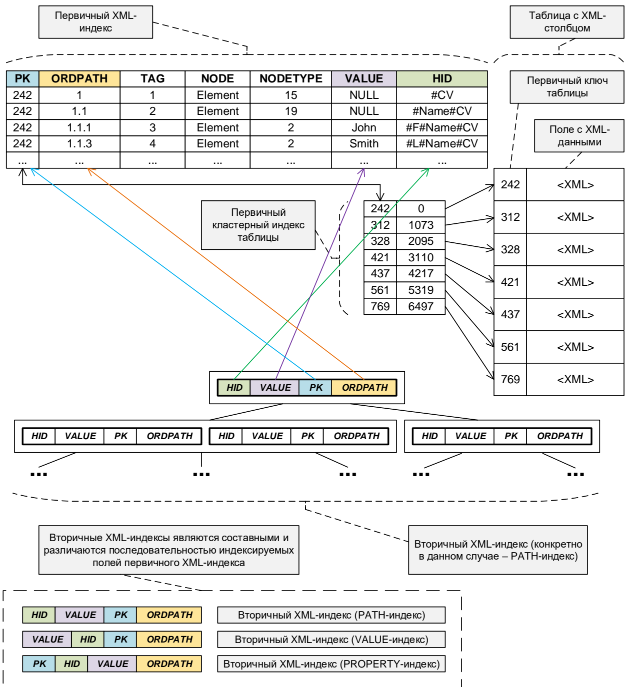
Рисунок 2.4.u — Схематичное представление XML-индекса
