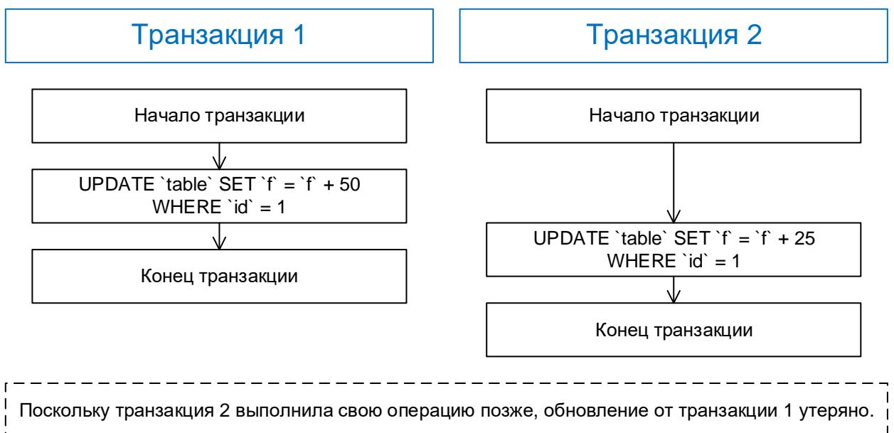
Рисунок 5.5.c — Потерянное обновление
