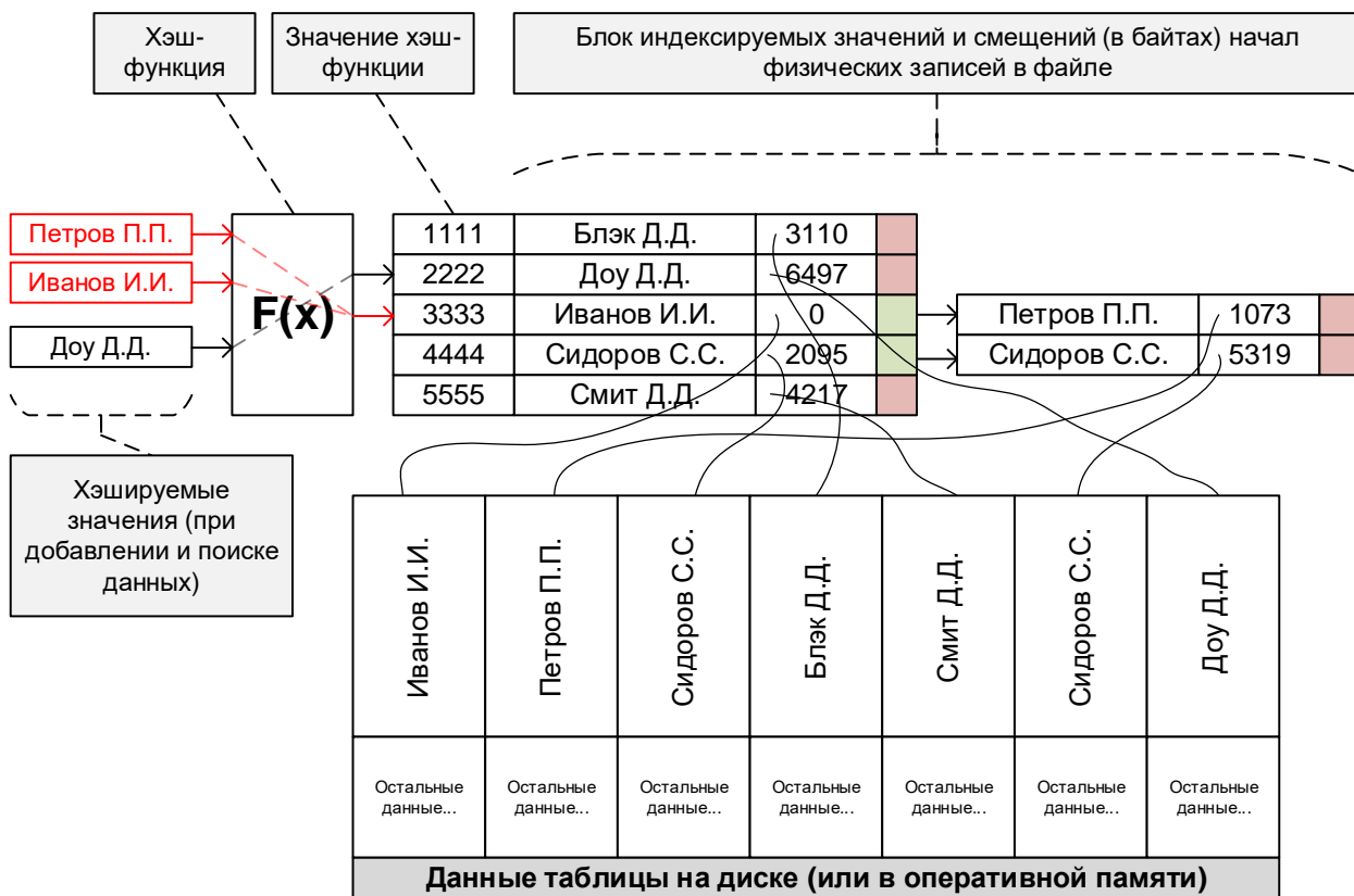
Рисунок 2.4.l — Схематичное представление индекса на основе хэш-таблицы
