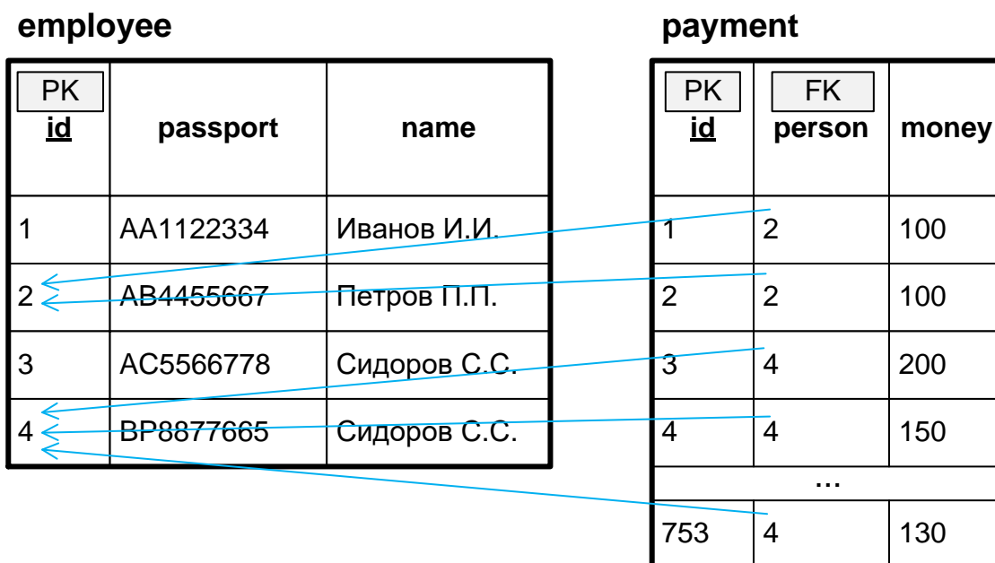
Рисунок 2.2.l — Внешний ключ
