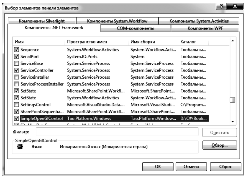
Рис. 9.4. Добавление компонента
