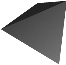
Рис. 8.1. Тетраэдр (3,3)
