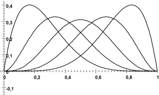
Рис. 3.2. Многочлены Бернштейна
