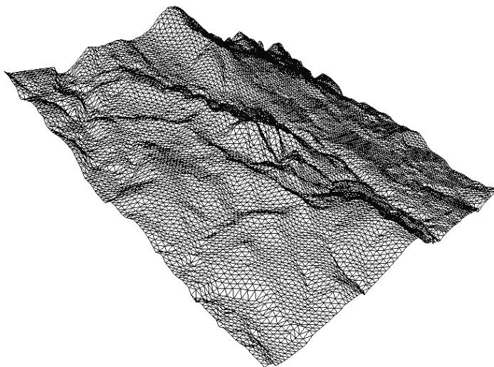
Рис. 9.17. Поверхность, заданная таблично
