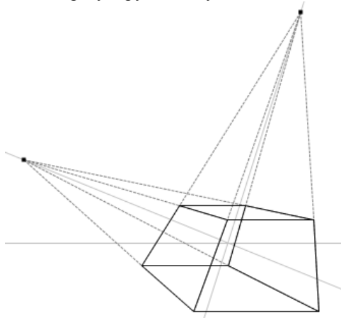
Рис. 8.12. Двухточечное проецирование
