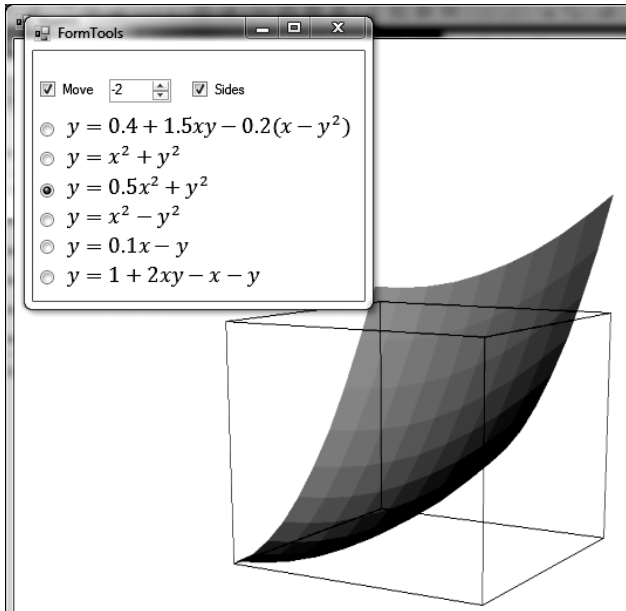
Рис. 6.3. Поверхность z=1+2*x*y-x-y в единичном кубе
