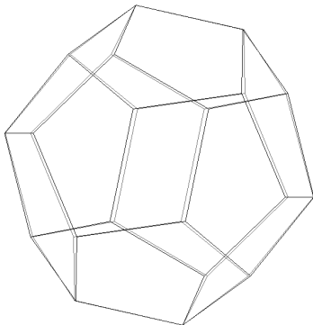
Рис. 8.13. Стереорезультат многогранника
