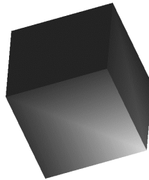
Рис. 8.2. Куб (4,3)
