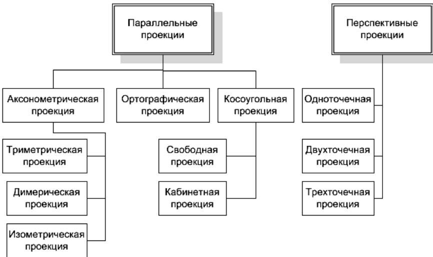
Рис. 3.7. Виды проецирования
