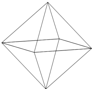
Рис. 8.7. Октаэдр
