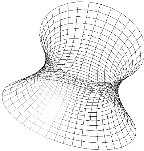
Рис. 9.16. Однополостной гиперболоид
