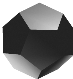
Рис. 8.5. Додекаэдр
