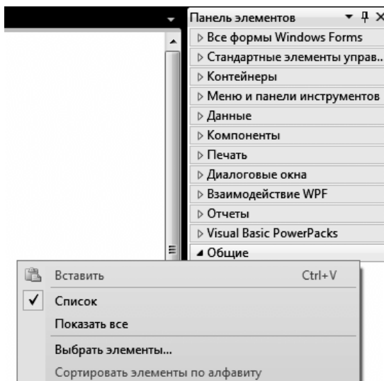
Рис. 9.3. Выбор элементов
