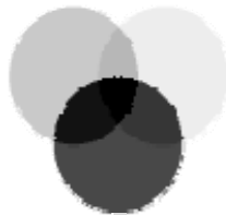
Рис. 2.23. Модель CMY
