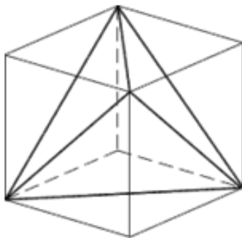
Рис. 8.6. Построение тетраэдра
