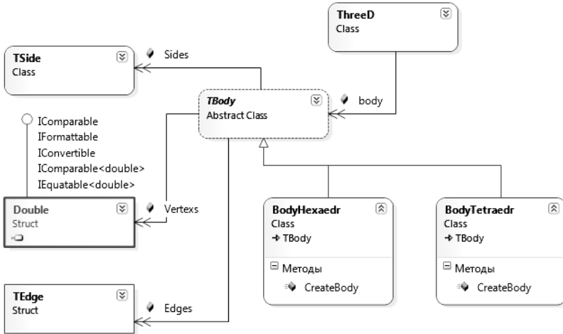
Рис. 3.15. Диаграмма классов
