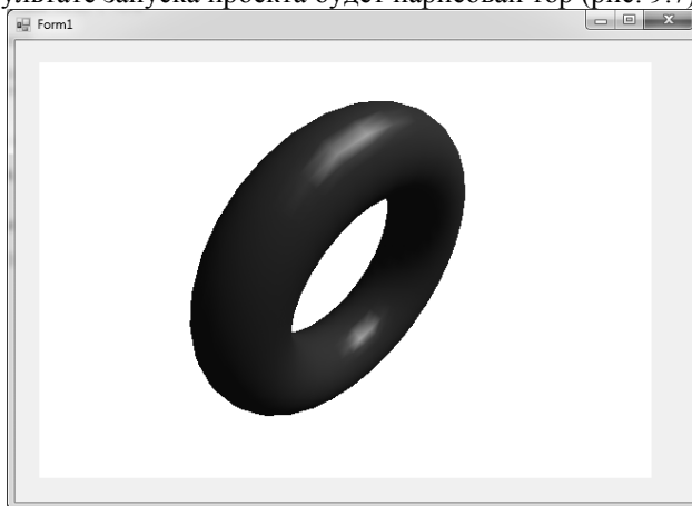
Рис. 9.7. Тор
