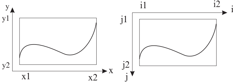
Рис. 5.4. Масштабирование графиков
